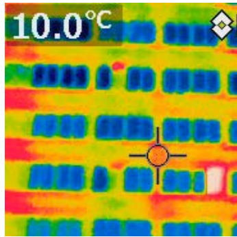
Thermographie de la façade ouest.
